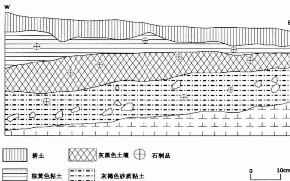
图 2 桃山遗址地层剖面图 Fig.2 Stratigraphic profile of the Taoshan site
