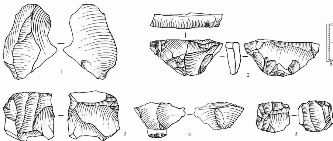
图 6 第 2 层石制品
