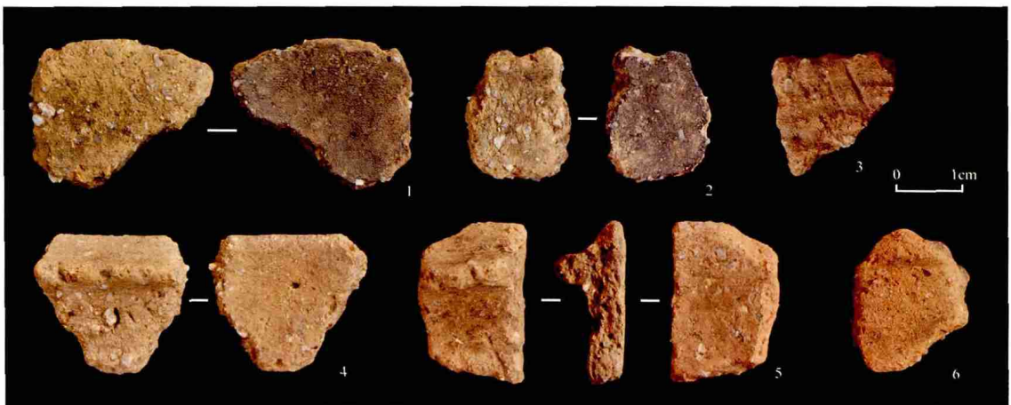
图 7 第 2 层陶片
