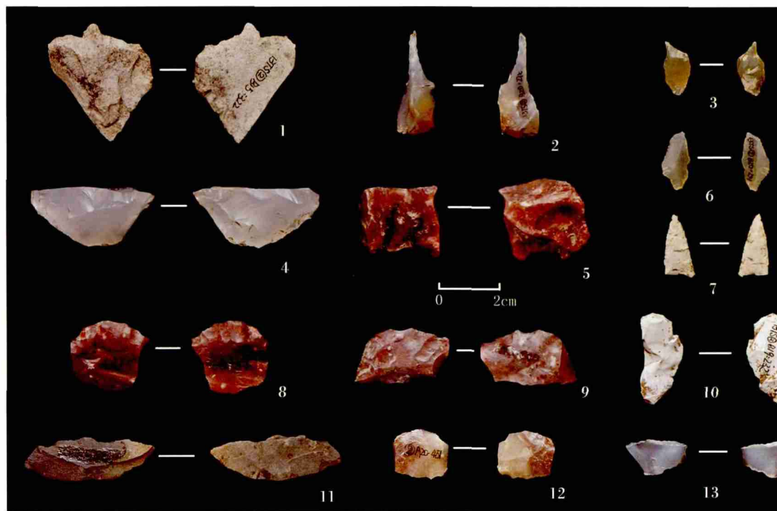
图 5 第 2 层石制品
