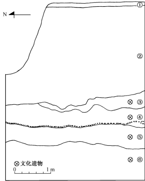
图 3 三棵树遗址东壁地层示意图
