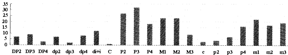
图 1 田园洞大中型哺乳动物牙齿统计柱状图
