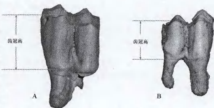
图3 牙齿齿冠测量方法
