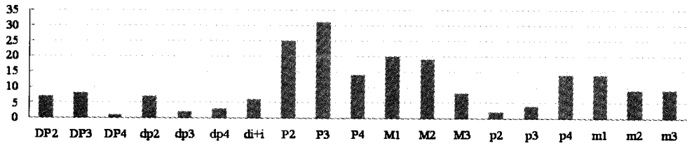
图 2 田园洞梅花鹿牙齿统计柱状图
