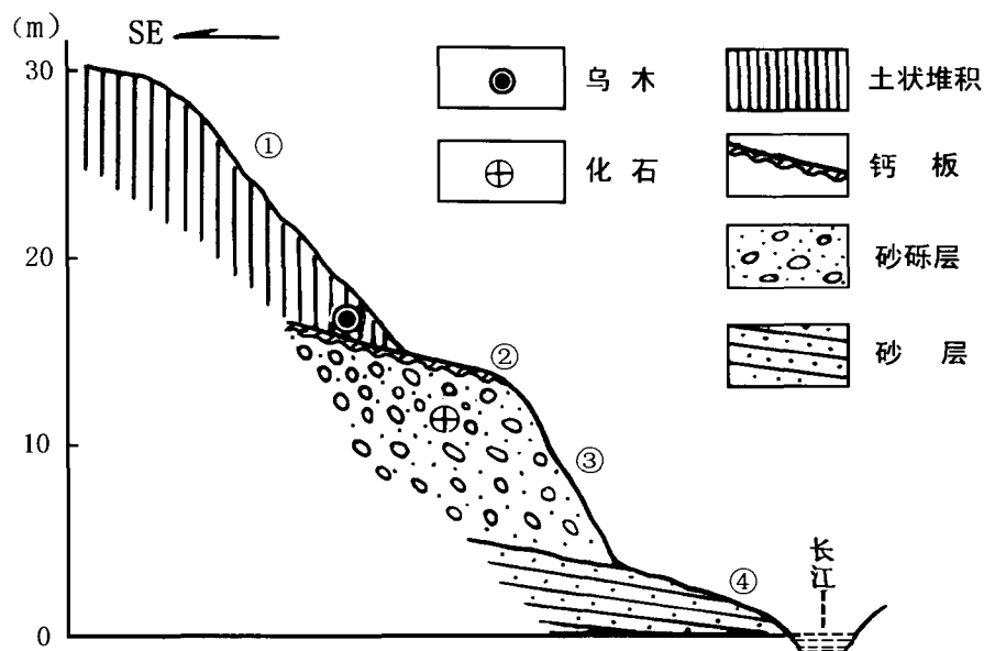
图 2 综合地质剖面图 General strata section of the site
