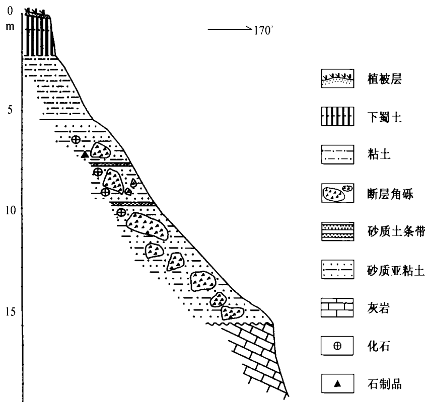
图 2 金盆洞旧石器地点地层剖面图
