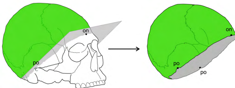
图1 本文使用的头盖部面积的测量方法
