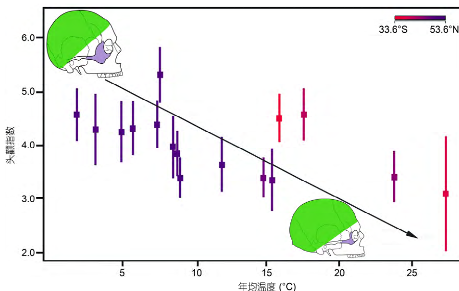
图5 头颞指数的纬度分布特点及与温度的关系
