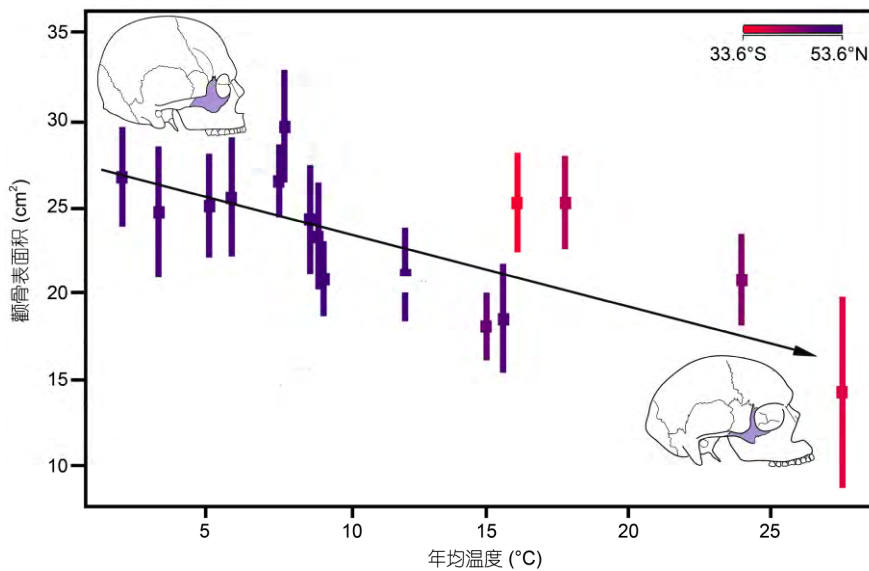
图4 颧骨表面积的纬度分布特点及与温度的关系
