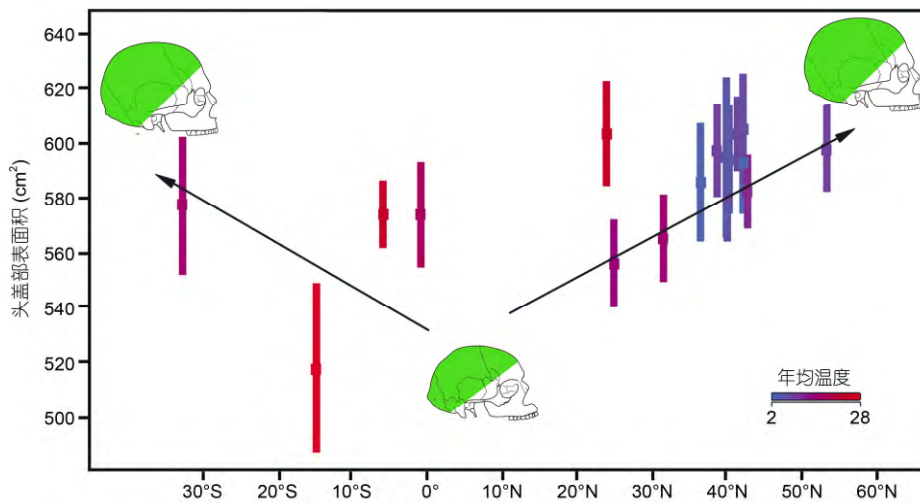
图3 头盖部表面积的纬度分布特点及与温度的关系
