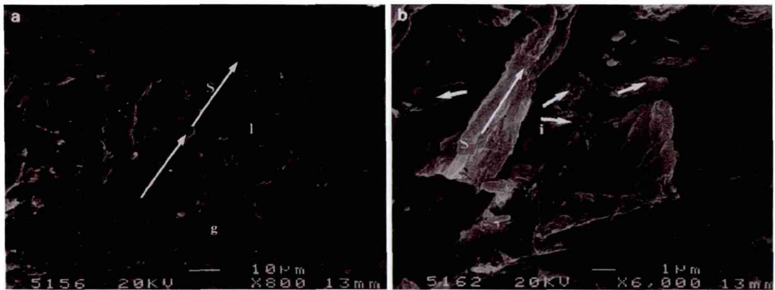
图 4 ×800 (左) ×6000 (右) 牙齿珐质三维微观结构电镜扫描图像 [13]
