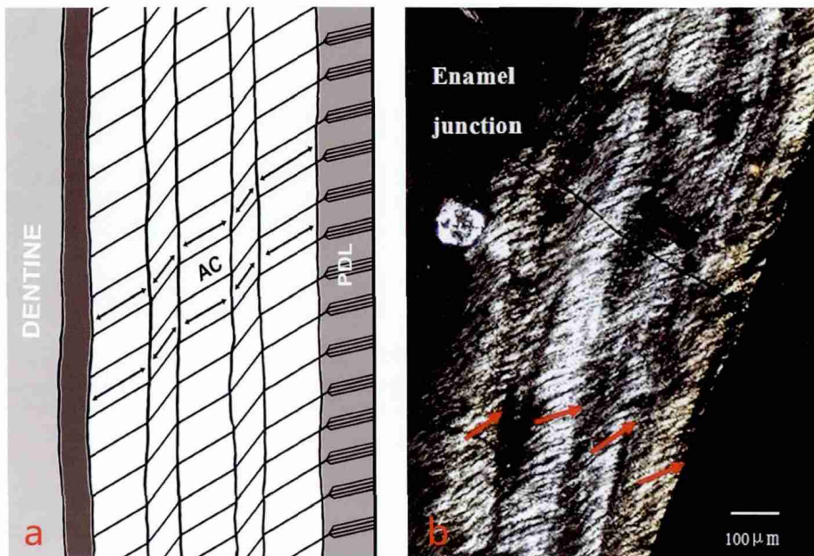
图3 牙齿珐质中胶原纤维方向示意图
