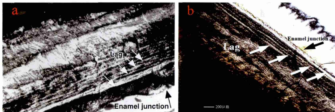
图 2 现代普通马 [12] 与许家窑遗址出土普氏野马垩质切片对比图
