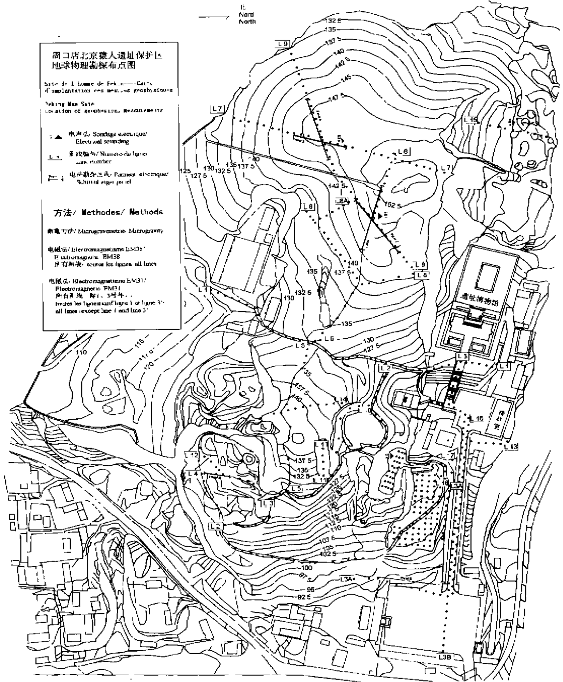
图 1 周口店遗址保护区地球物理勘探布点图 Frame work of the geophysical measurements
