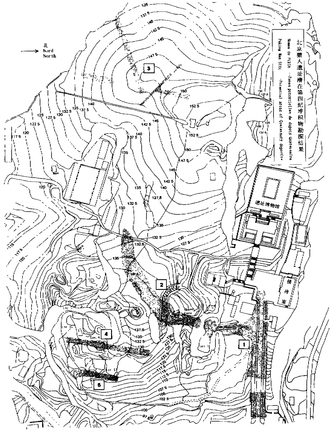
图 3 周口店遗址保护区内潜在第四纪堆积物勘探结果(阴影区) Potential areas of Quaternary deposits
