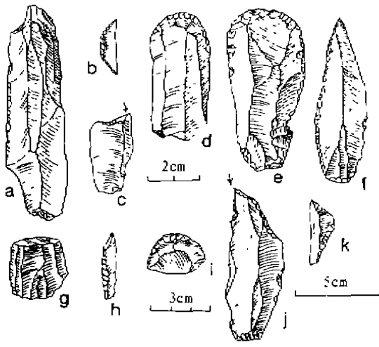
图 7 模式IV技术。北非和东非晚期石器时代的石制品。出自 Gobedra 遗址(埃塞俄比亚) (a) 修整石叶; (b) 月形器, Eburran 工业(肯尼亚); (c) 雕刻器; (d) 端刮器, Ibero-Maurusian 工业(摩洛哥); (g) 两端剥片的细石叶石核; (h) 钝背细石叶; (i) 短身端刮器, Capsian 工业(突尼斯); (e) 端刮器; (f) 钝背石叶; (j) 雕刻器, (k) 细石器。(依 Brooks, 1988d)
