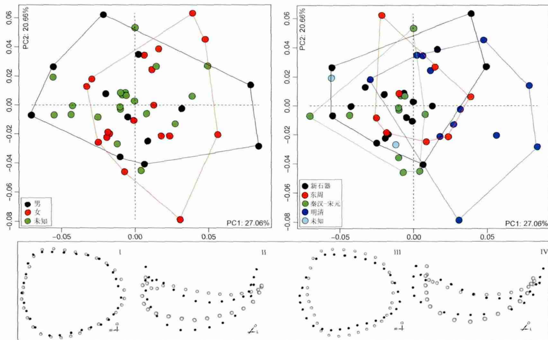
图 5 上颌第四前臼齿的主成分分析
