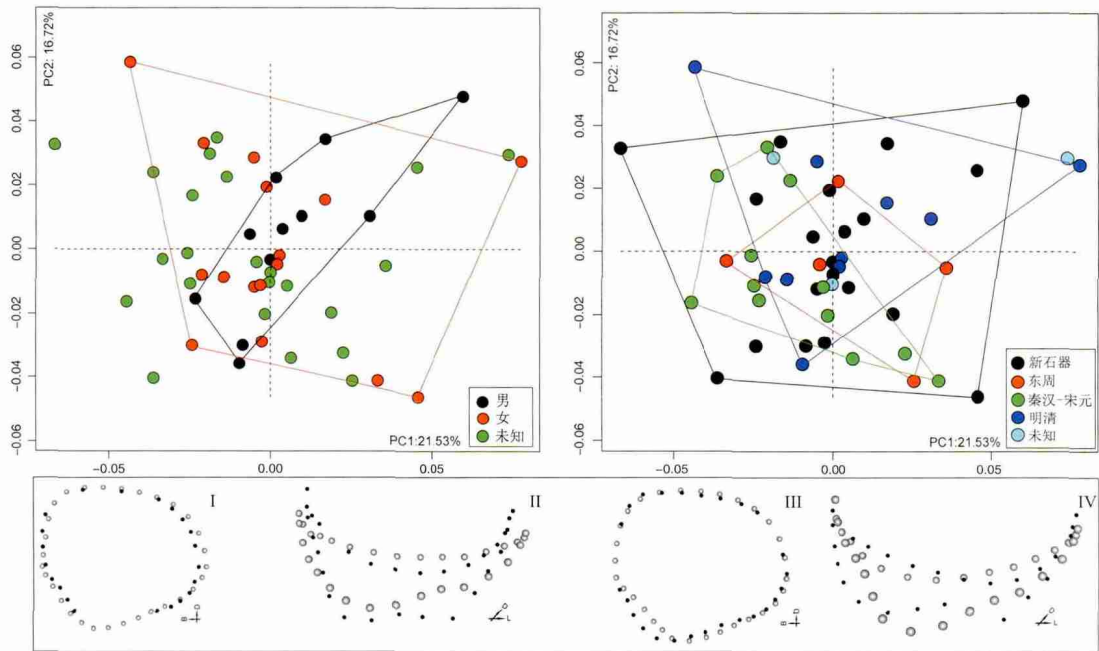
图 3 上颌第三前臼齿的主成分分析
