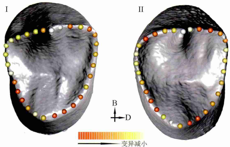
图 2 上颌第三 (I)、四 (II) 前臼齿 EDJ 的平均形状和不同位置的变异大小
