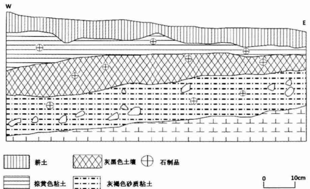
图 2 桃山遗址地层剖面图 Fig.2 Stratigraphic profile of the Taoshan site
