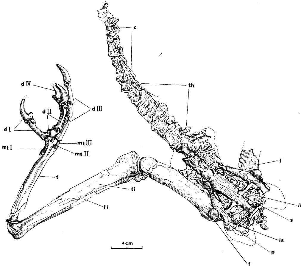
图 1 泰山齐鲁鸟(新属种)的正型标本(IVPP V 12351), 腹、侧视
